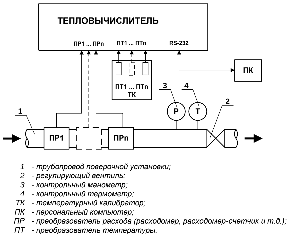
Рис.Г.1. Схема подключения ТСч при поверке методом непосредственного сличения.
